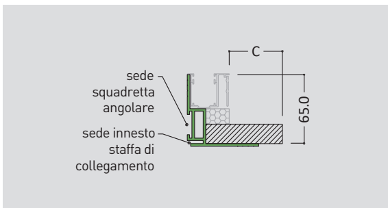
APPLICAZIONE CON BATTUTA INVERTITA
