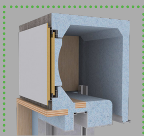
Ispezione Frontale
