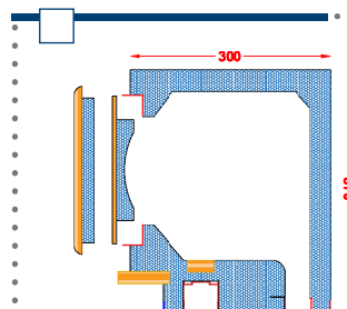
Ispezione frontale infisso filo muro interno con incasso zanzariera
