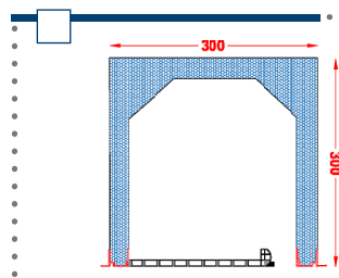
Celino in PVC infisso filo muro interno
