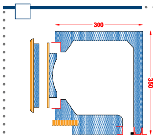
Ispezione frontale infisso filo muro interno
